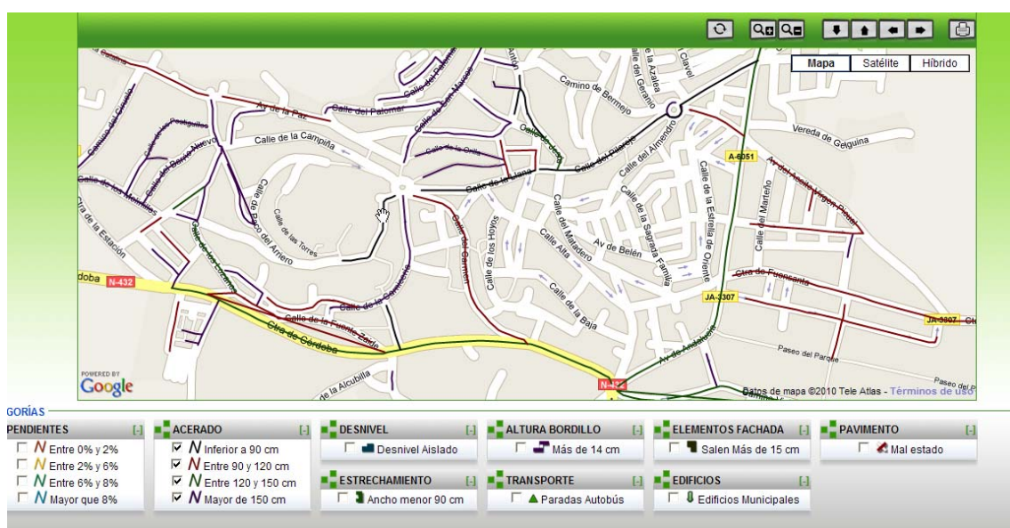
Ejemplo de callejero con el ancho de acerado representado
